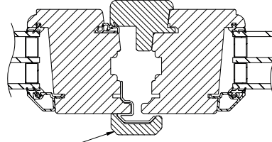
Horizontalsnitt pardörr
